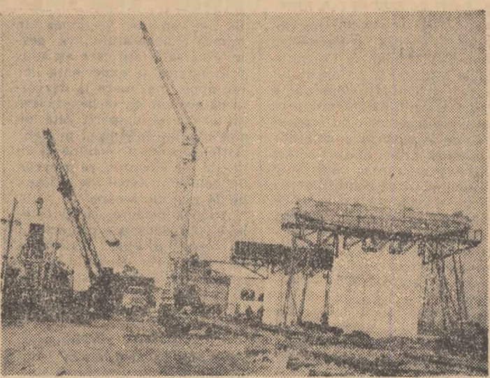
La viitorul viaduct de acces de la Giurgeni unde se construiește un pod peste Dunăre. Macarale de mare tonaj sînt folosite la turnarea grinzilor prefabricate.
