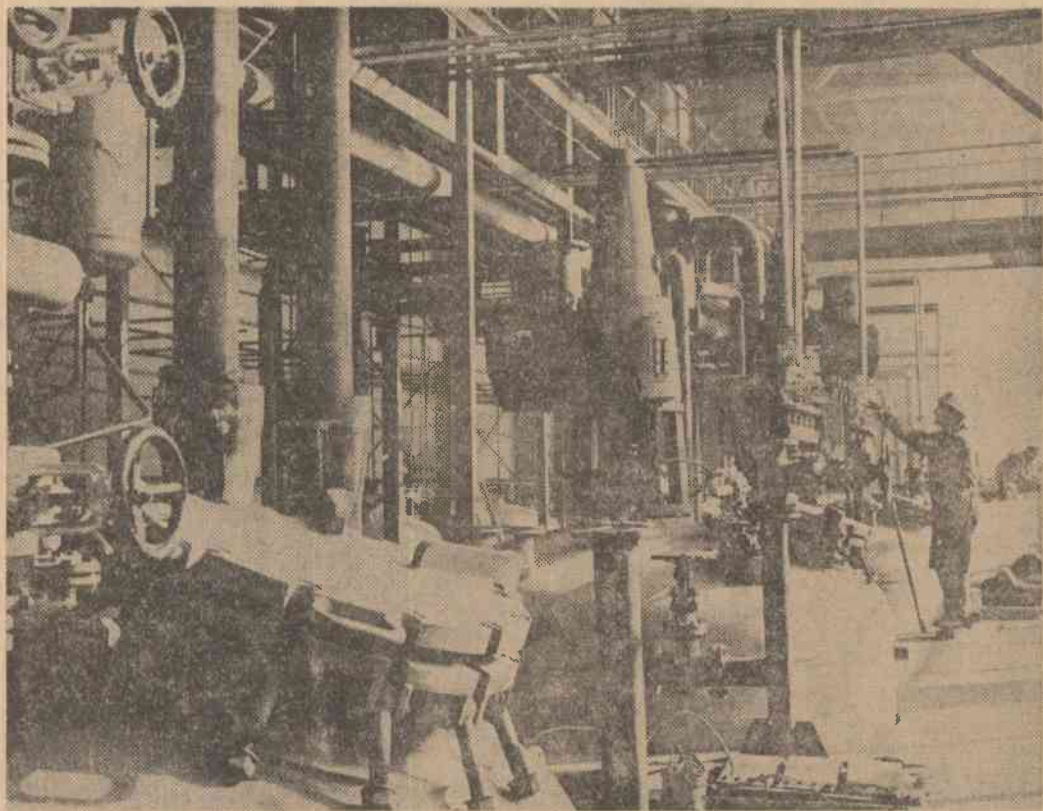
Stadiul avansat al lucrărilor de montaj de la Combinatul chimic din Rîmnicu Vilcea vestește prima recoltă... chimică, care se va obține aici în anul viitor. În clișeu: Instalația de polimerizare din cadrul fabricii de cristalizare a sării. Foto: AGERPRES
