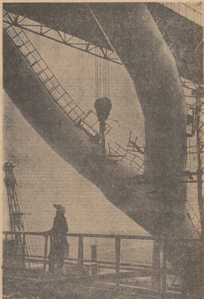
În imaginea de mai sus vă prezentăm furnalul de 1700 mc., unul din primele obiective ale gigantului siderurgic de la Galați. De curînd aici au început lucrările unei alte importante capacități — laminorul de benzi la cald, care va intra în funcțiune în a doua jumătate a anului 1969.
