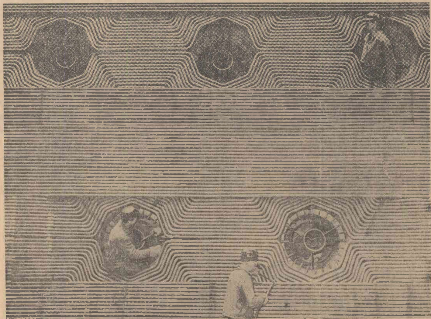
În cadrul noii etape de dezvoltare a Centralei electrice și de termoficare — Borzești, lucrările la cel de-al doilea cazan oferă în aceste zile o imagine care la prima vedere surprinde. Desenul perfect trasat ca pe o coală de calic, nu reprezintă altceva decât țevăria din camera focarului căruia sudorii îi execută îmbinările Foto: NICU VASILE
