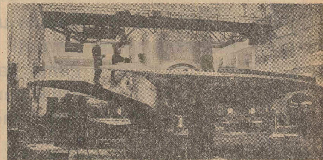
La Uzina de produse metalice „Al XXII-lea Congres al P.C.U.S.” din Leningrad a fost realizată a treia turbină de apă pentru hidrocentrala de la Saratov. Unul din principalele ansambluri ale mașinii — rotorul — cu un diametru de peste 10 m. cu palete rotative, a trecut probele necesare. În clișeu — Rotorul turbinei pentru hidrocentrala de la Saratov.
