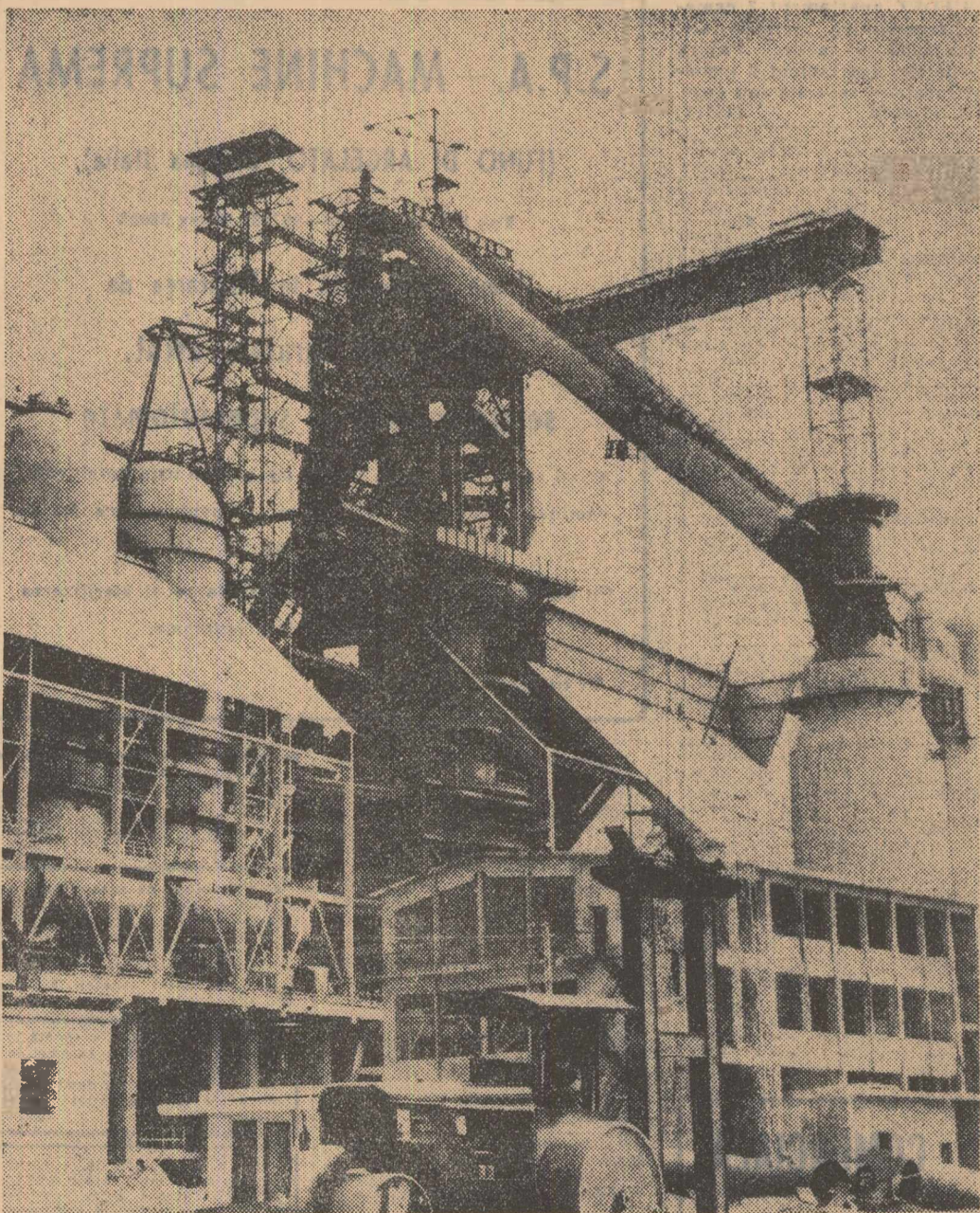
La Combinatul siderurgic „Gh. Gheorghiu-Dej” din Galați se apropie intrarea în funcțiune a primului furnal. Acesta este proiectat la o capacitate de 1 700 mc, fiind cel mai mare agregat siderurgic de acest fel din țară. În momentul de
