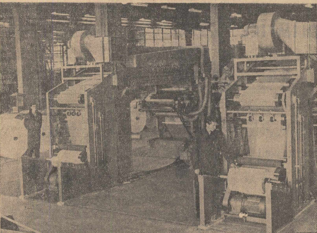
La Fabrica pentru prelucrarea maselor plastice din orașul Iași, zilele acestea a intrat în probe tehnologice o nouă linie de fabricație care va produce pe scară industrială saci din polietilenă pentru agricultură. În foto: Noile mașini de imprimat cu o capacitate de 3.000 buciți pe oră
