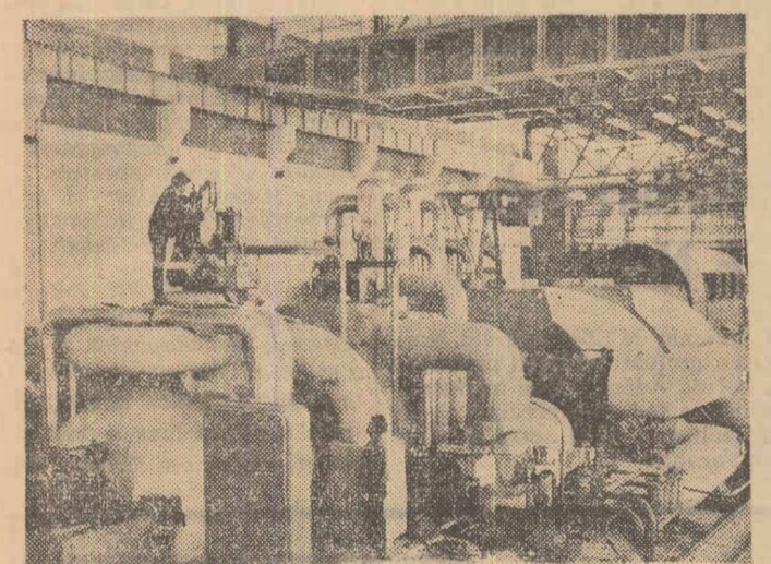
La Centrala electrică de termoficare Craiova în timpul probelor turbinei de 315 MW.
