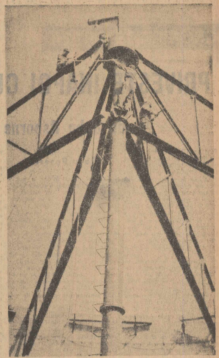
Pe șantierul rafinării din Pitești se află în curs de montare primul rezervor de 10.000 mc pentru produse petroliere. În cliseu: Membrii echipei condusă de Tănase Negoi, de la întreprinderea montajă București, montează semifermele de la capacul rezervorului. Foto: NICU VASILE
