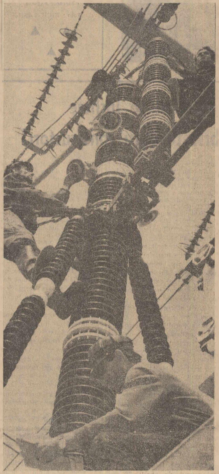
Din agitația involburată a apelor Argeșului se nase acum megawații cărbunelui alb. Înainte de a intra în sistemul energetic național ei trec prin stația de interconectare de 220 KW. Activitatea de întreținere a acestor stații necesită o grijă și o atenție deosebită. În imagine: se lucrează la întreținerea echipamentului de înaltă tensiune.
