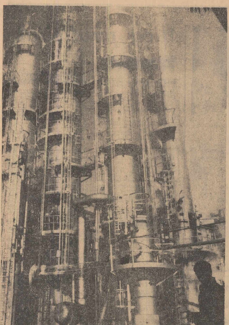
Aspect parțial al instalațiilor de solvare a motorinei de la rafinăria din orașul Gheorghe Gheorghiu-Dej
