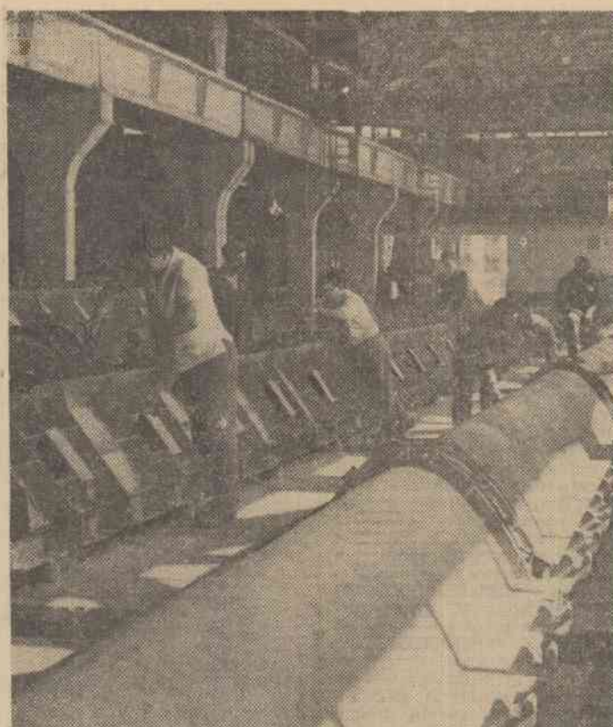
Două aspecte de pe șantierul Întreprinderii de prefabricate Călărași: În stînga, sectorul tiparelor metalice pentru fabricarea igheburilor; în dreapta, impunătoarea estacadă de la depozitul de agregate Foto: AGERPRES
