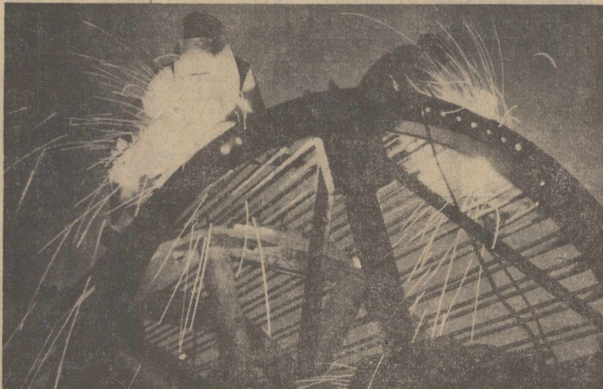
Anul acesta, constructorii de pe șantierul podului de peste Dunăre, au între altele sarcina să termine așezarea pilelor-culee pentru fundații de pe cele două maluri ale fluviului. Datorită măsurilor luate pentru introducerea unor metode avansate, lucrările se desfășoară într-un ritm viu. În cliseu: Un aspect de la sudarea carcascilor metalice necesare coloanelor de beton armat pentru fundații.
