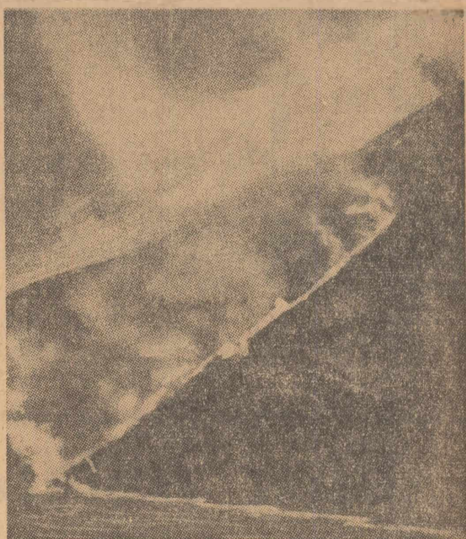
În ultimele zile vulcanul Stromboli din Sicilia, și-a intensificat erupția, aruncînd spre cer puternice suvoaie de lavă și pietre. În fotografia de mai sus, o impresionantă coloană de lavă incandescentă coboară spre mare.
