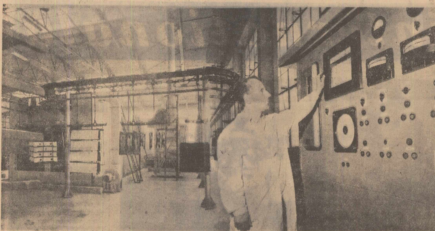
Prin punerea în funcțiune a noii secții de emalaj de la întreprinderea „1 Septembrie” din Satu Mare, procesul de fabricație a mașinilor de gătit cu gaze s-a îmbunătățit substanțial. În clădire: Maistrul Ilie Păruș urmărește, la panoul de comandă, funcționarea cuptorului tunel
