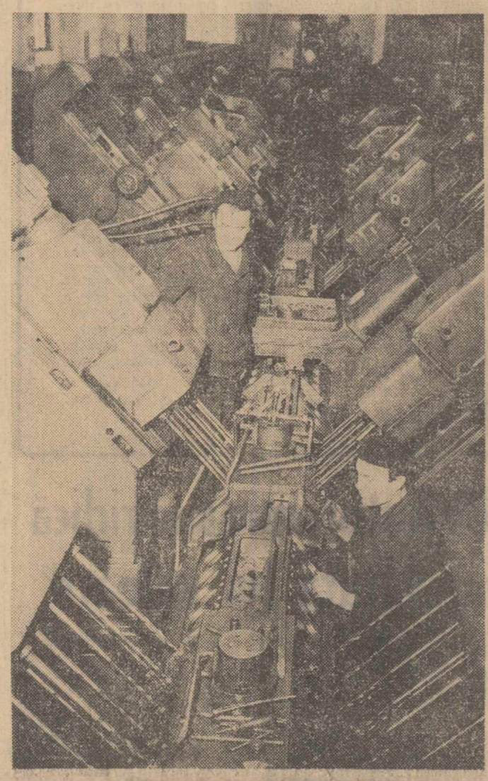
Aspect al liniei de prelucrare a blocului motor de la uzina „Steagul roșu” Brașov
