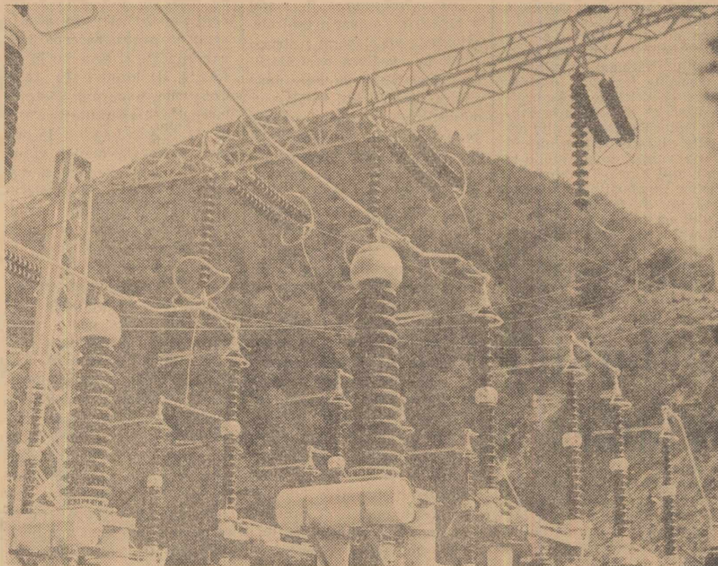
Înainte de a porni pe magistralele aeriene ale țării, fluviul de lumină produs de apele Argeșului în centrala subterană trece prin stația de transformare.
