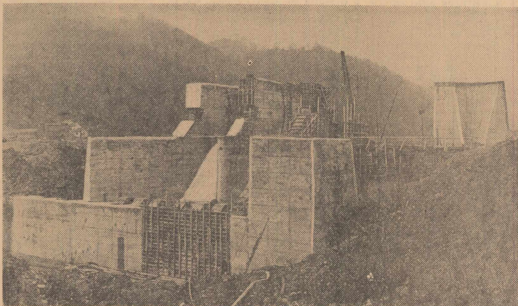
Apele Argeșului și ale afluenților săi, după călătoria prin „galeria de fugă” și transformarea în energie electrică vor fi puse din nou la treabă odată cu terminarea construcției celor patru microhidrocentrale, în aval de centrala electrică (în afara celor în amonte de barajul Vidraru). Iată unul dintre „puii” care cresc, în prezent, cu repeziune: microhidrocentrala Oiești.
