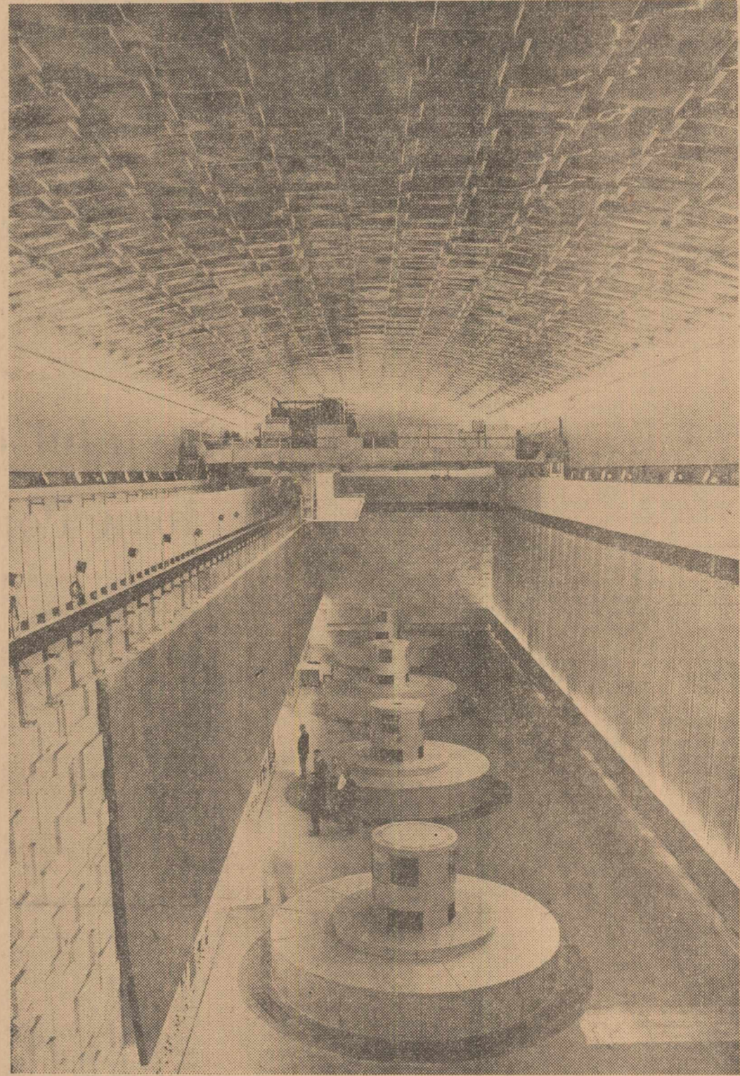
„Palatul subteran” așa cum arăta la 9 decembrie 1966!
