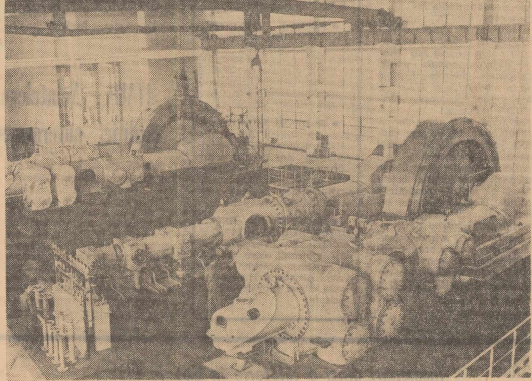
La Combinatul chimic din Făgăraș a fost montat și dat în exploatare cel de-al doilea compresor de mare capacitate, necesar fabricii de amoniac. În cișcu: Vedere din sala compresoarelor
