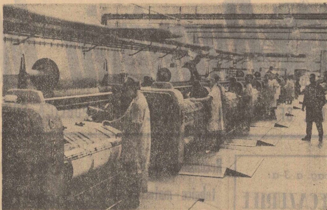
La întreprinderea „Munca Textilă” din București a fost introdusă o nouă tehnologie de fabricație: textilele nețesute. În colaborare cu Institutul de cercetări textile, colecțivul fabricii a realizat, pe baza acestei tehnologii o seamă de sortimente de articole de consum și de uz industrial. În clădire: aspect dintr-una din sălile de fabricație unde se realizează noul sortiment
