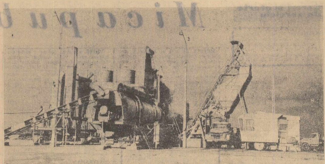
Instalație modernă de mixturi asfaltice și beton asfaltic folosită la asfaltarea străzilor Capitalei. Într-o oră se pot asfalta 20 de tone. Calitatea lucrului efectuat este socotită ca foarte bună. Foto: FLORIN ȘTEFĂNESCU
