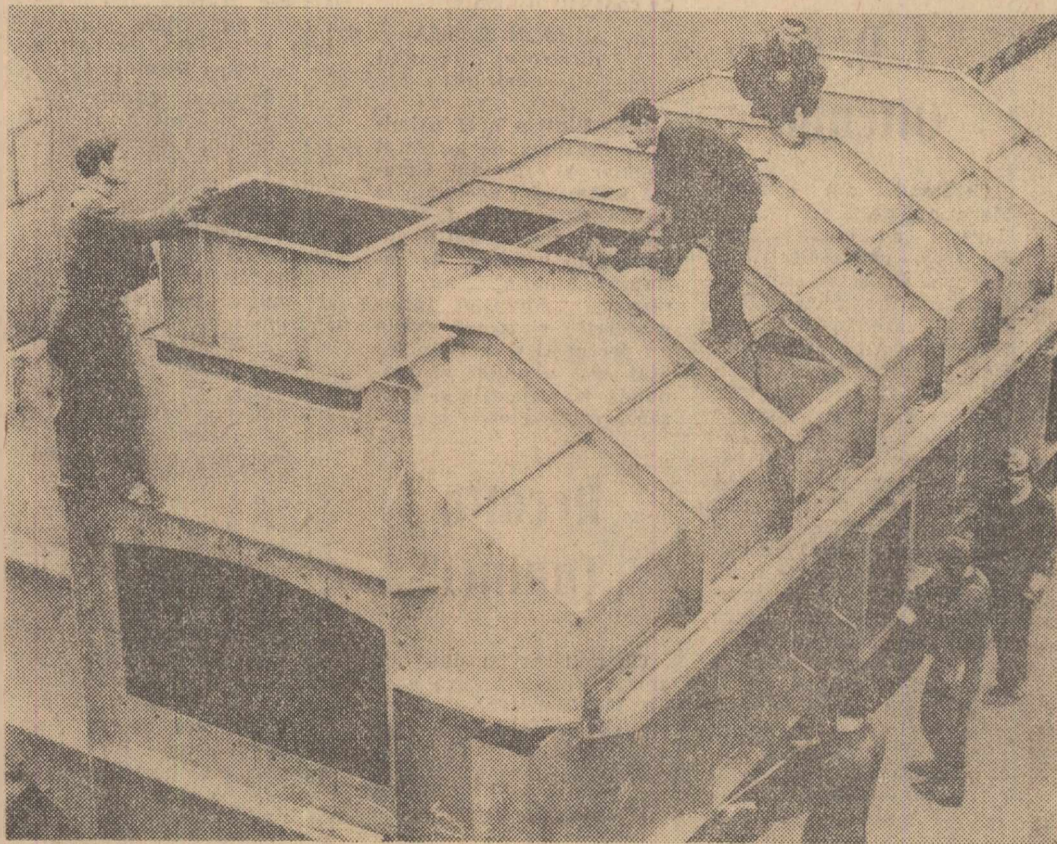
Cazangii din brigada lui Mircea Voronca execută ultimele finisări la cupțorul destinat Uzinei de aluminiu din Slatina
