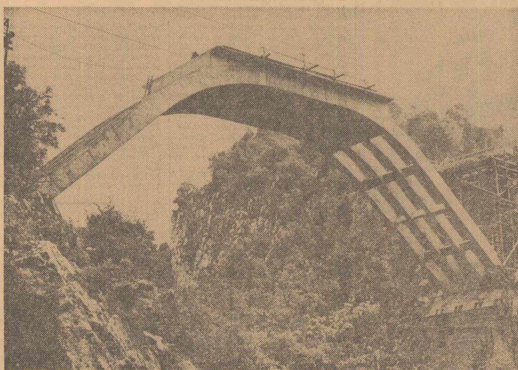
Bolta celui mai înalt viaduct din țară construit pe drumul Petroșani-Simeria a fost recent decroșată. În prezent se montează traversele care vor completa această impresionantă lucrare Foto: FLORIN ȘTEFĂNESCU
