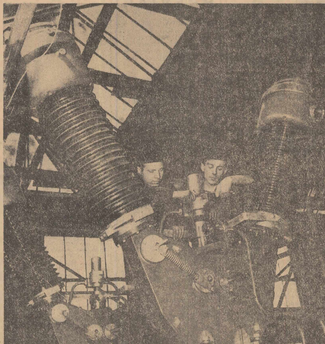
Printre produsele binecunoscutelor uzine craiovene „Electroputere” se numără, de curînd, și interupătorul de 110 KV-1600 A-6000 MVA destinat rețelelor electrice de înaltă tensiune. În clipă: montorii Luca Ion și Constantin Velicu lucrînd pe standul de probă la reglarea noului produs
