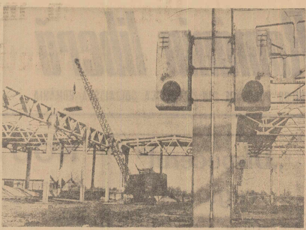
La Tecuci se construiește o hală de 1600 m.p. din prefabricate, rezervată pentru reparații și revizii auto. În clișeu: Aspect de pe san țier. Cu ajutorul macaralei se ridică o placă de planșeu
