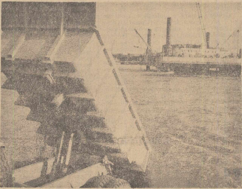
Aspect din timpul construcției digului amonte pe șantierul sistemului hidroenergetic și de navigație „Porțile de Fier”
