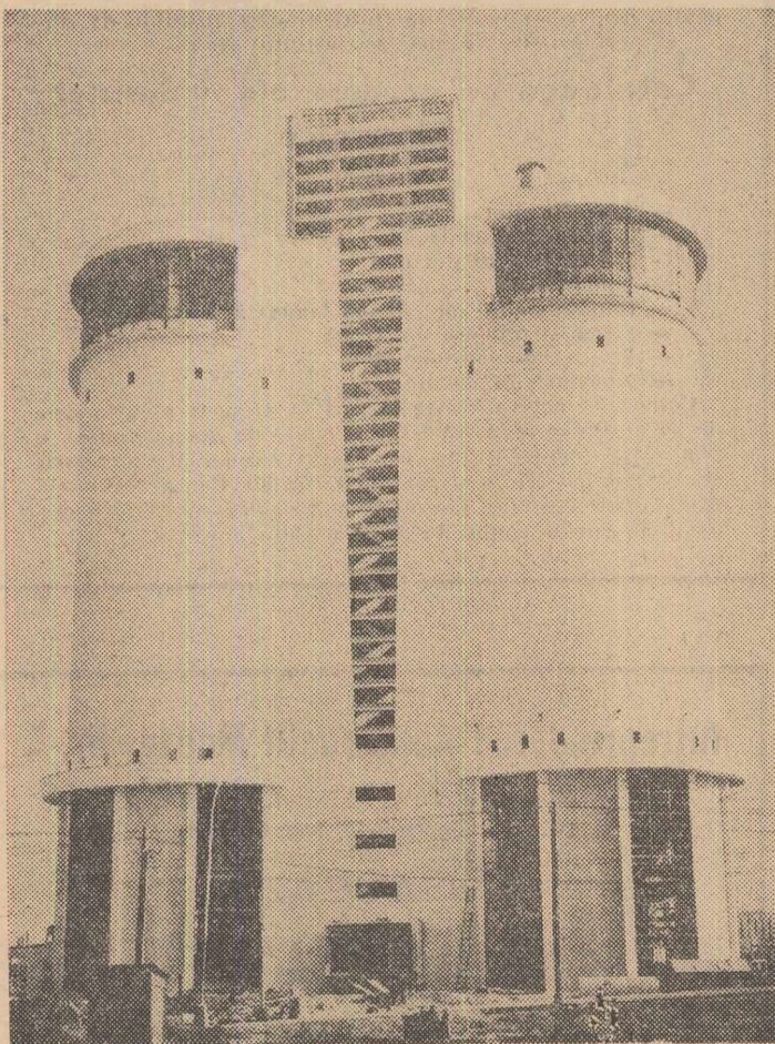
Industria noastră chimică, în 1970, va pune la dispoziția ogoarelor patriei peste 1.100.000 tone îngrășăminte substanțiale activă. La realizarea acestei sarcini își aduce contribuția și tînărul combinat de îngrășăminte azotoase de la Tg. Mureș. În clișeu: turnurile de granulare a azotatului de amoniu
