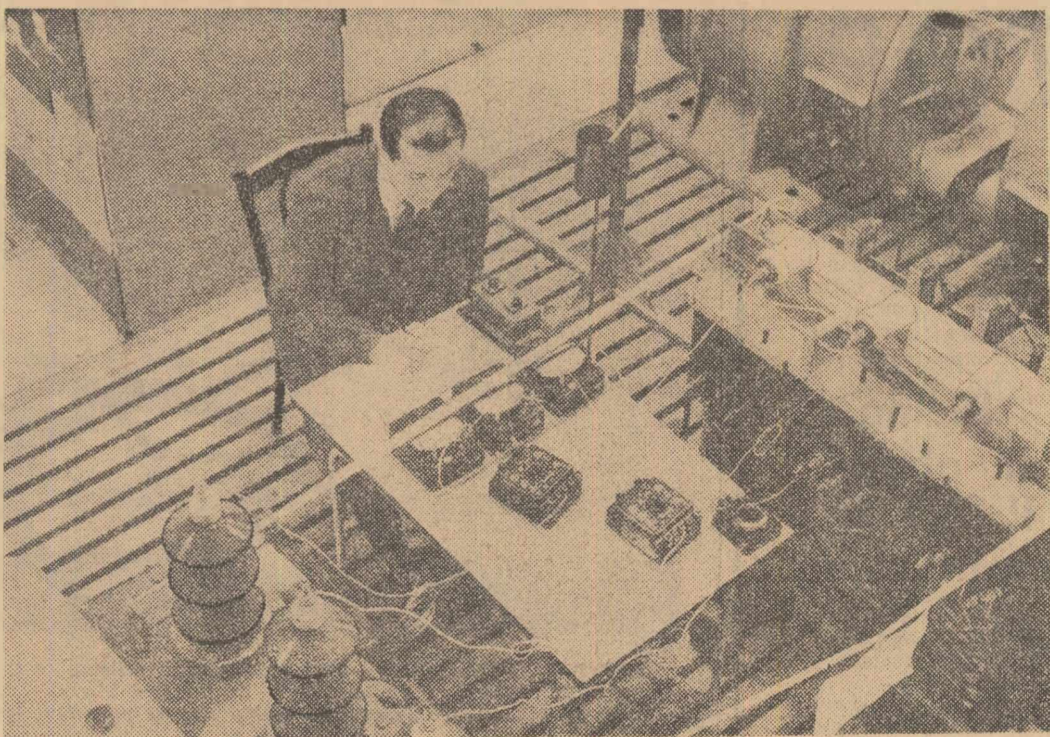
În laboratorul de mașini și transformatoare al Institutului de cercetări și proiectări pentru industria electrotehnică din București. Fotografia a fost luată în momentul executării unor încercări de încălzire la prototipul de transformator cu înfășurări din conductori de aluminiu izolați cu email
