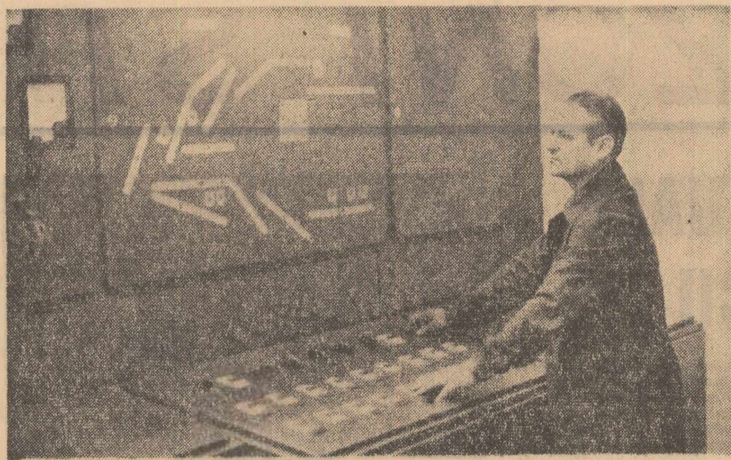
Uzina „Înrîțirea” din Oradea — care fabrică mașini-unele cunoscute și apreciate atît în țară cît și peste hotare — continuă să se dezvolte, sporindu-și capacitatea de producție. Printre lucrările realizate se numără și noua turnătorie, de unde vă prezentăm tabloul de comandă.
