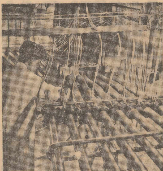
Institutul de energetică al Academiei Republicii Socialiste România. În laboratorul de modelare a proceselor de ardere din focare ciclon pentru combustibili solizi se urmărește ridicarea curbelor de viteze.
