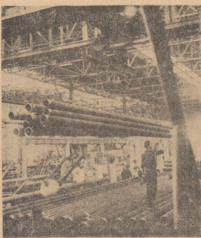
Uzina de ţevi din Roman. Paturi de depozitare a ţevilor în hala de tras la rece
