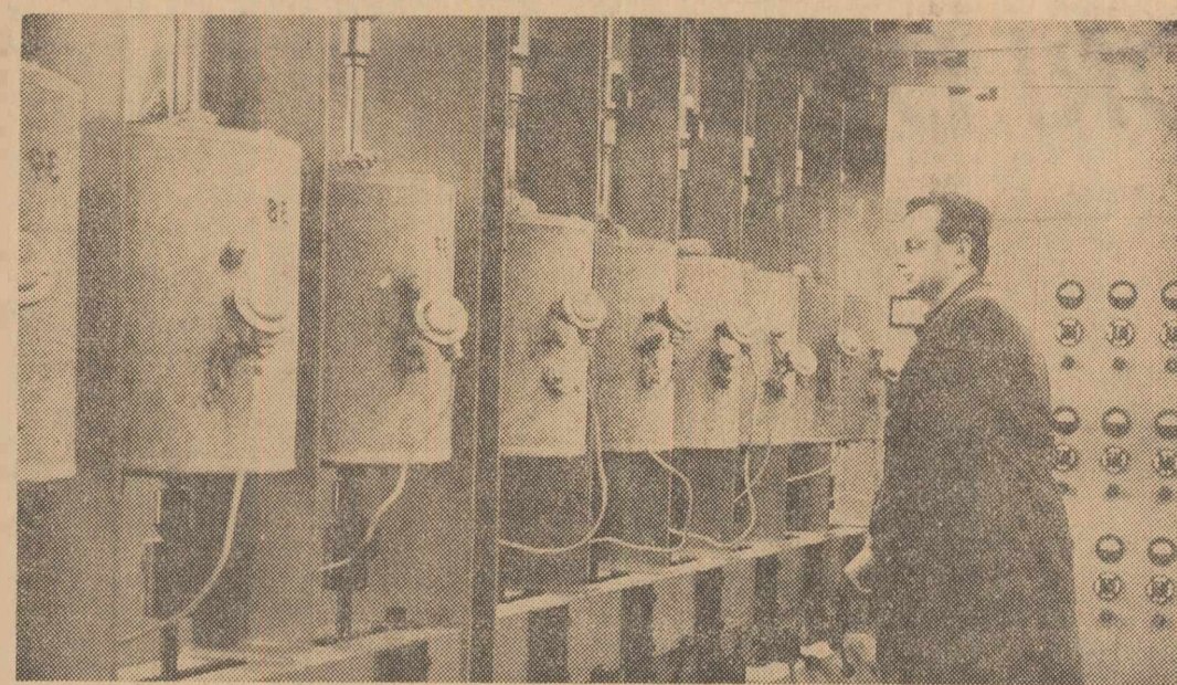
Laboratorul de încercări de fluaj de la Institutul de cercetări metalurgice din Capitală: aici se determină proprietățile de fluaj la temperaturi ridicate ale oțelurilor
