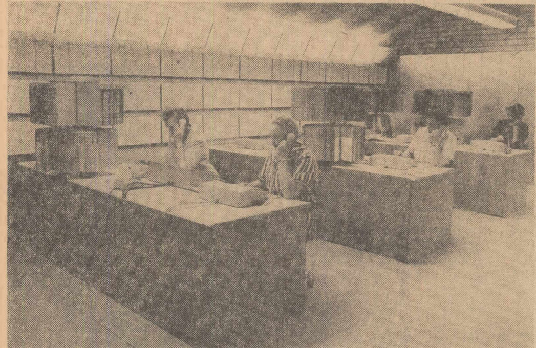
În Finlanda funcționează, de curînd, unul din cele mai moderne sisteme telefonice pentru căile ferate, din lume. Caracteristic pentru acest sistem automat, generalizat în prezent în întreaga țară, este marea viteză cu care sînt transmise, spre receptor, numerele selectate. În fotografie: aspectul unuia din sălile centralei telefonice pentru căile ferate, din Helsinki.
