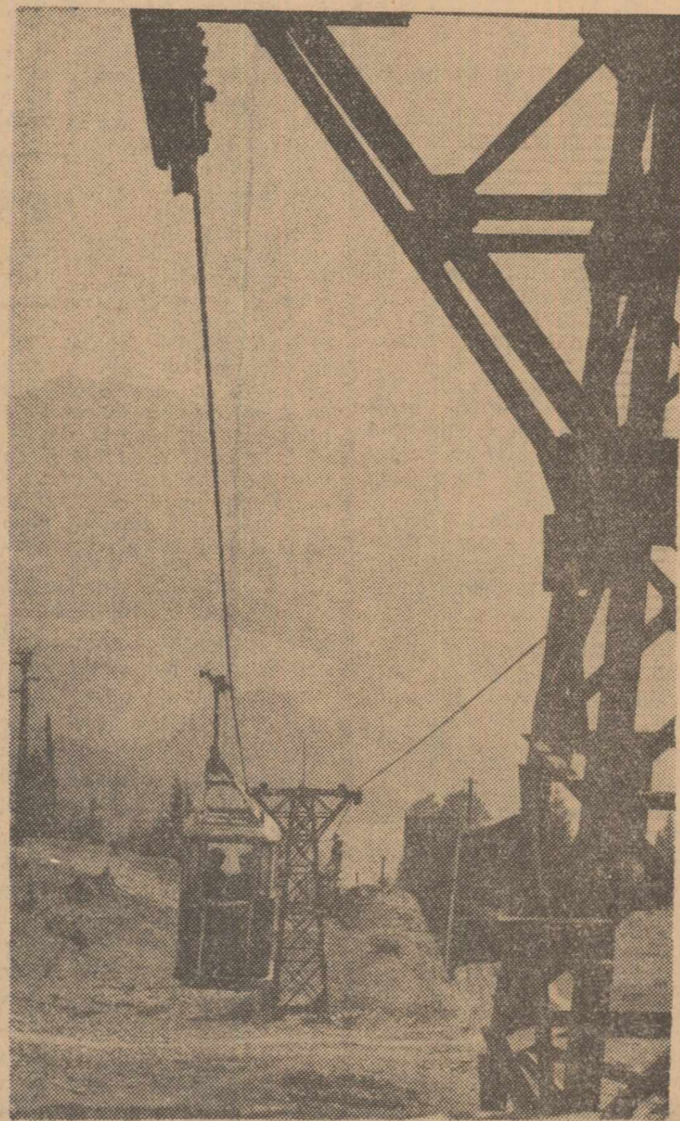
Fină acum transportul minerilor și al materialelor către mina Torioaga se făcea anevoios, exploatarea fiind situată la o altitudine de 1.400 m. Fină acum, pentru că recent s-a dat în folosință un teleferic în lungime de 2.100 m care leagă mina de Baia Borșa. În clișeu: Noul teleferic
