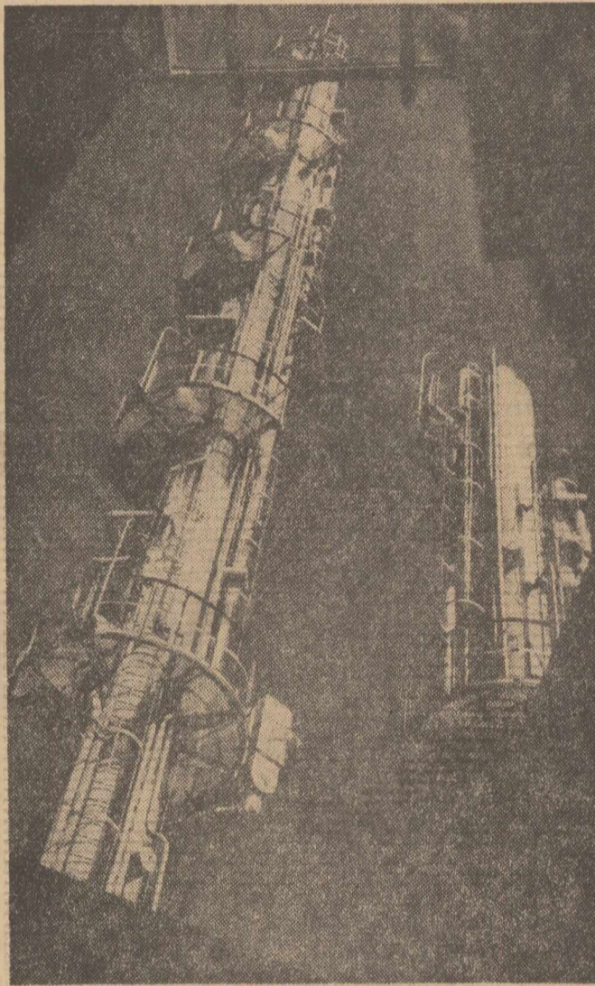
Una din instalațiile Combinatului petrochimic de la Brazi. Aspect de noapte
