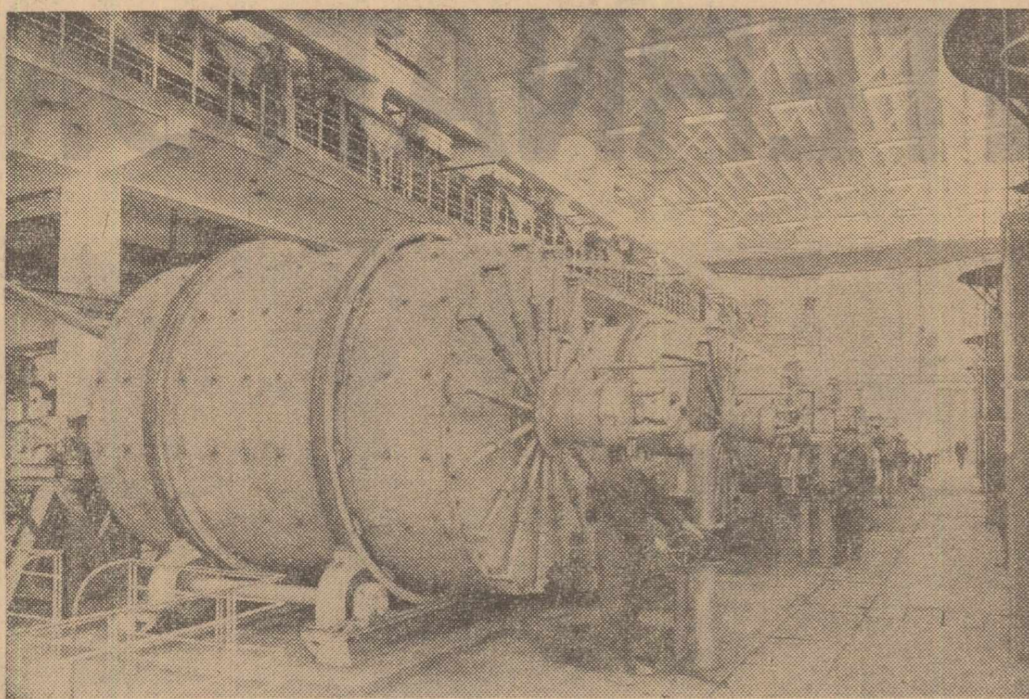
La Telieș a fost dată în folosință o uzină de preparare a minereurilor de fier din zăcămintele de la Telieș și Ghețar. Specialiștii de aici aplică pentru prima oară în țară metoda prășirii magnetizante și separarea magnetică pe cale umedă a minerului. Acest procedeu face să crească de două ori conținutul de fier al minerului. În clișeu. Aspect din sala filtrelor și separațiilor magnetice
