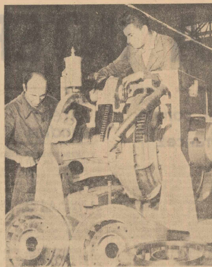
Printre ultimele realizări ale colectivului uzinei „Hidromecanica” din Brașov se află și convertizorul hidraulic de cuplu. Acest produs de înaltă tehnicitate, destinat tipurilor moderne de instalații de foraj fabricate de uzina „1 Mai” Ploiești, este proiectat de specialiștii ai Institutului de proiectări și cercetări utilaj petrolifer. În elieș: lăcătușii Petre Merth și Cornel Lăpăzan montează noul tip de convertizor.
