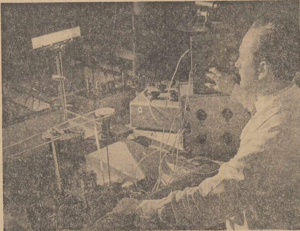
Fotografia noastră înfățișează laboratorul de curent continuu al Institutului de metrologie. Cercetătorul Radu Șovian efectuează etalonarea rezistențelor de valori mici, folosite în operația de transmitere a unității de rezistență de către centrele metrologice din țară către industrie.
