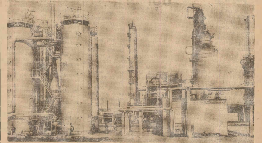
Instalațiile pentru producerea asfaltului la Rafinăria de ștei Mazovian de la Uzinele petrochimice din Plock (R.P. Polonă) care se află, în prezent, în construcție.
