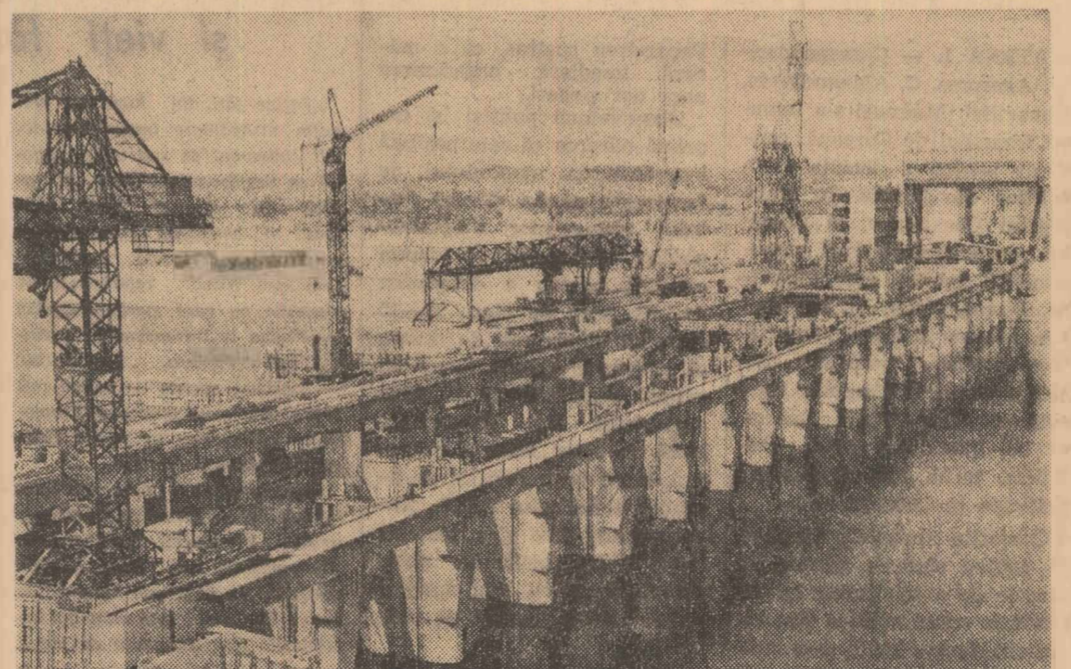
Aspect de pe șantiere de construcții al barajului noii hidrocentrale de lângă satul ucrainean Vișgorod, nu departe de Kiev — capitala R.S.S. Ucrainene.
