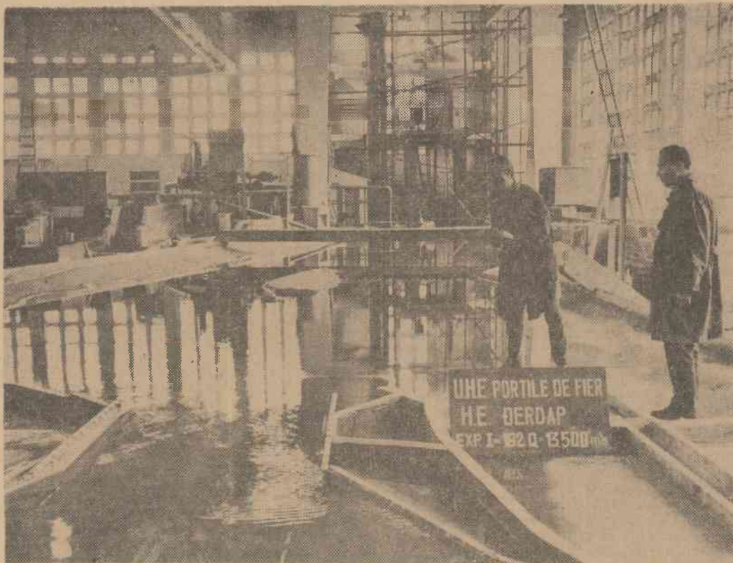
Înainte de a fi construite, marile obiective hidrotehnice sînt mai întîi „construite” la scară redusă. În laboratoare special amenajate, în care se creează condiții asemănătoare celor existente la scară naturală, modelele miniaturizate sînt experimentate, perfecționate, definite. Apoi, ele iau calea transunerii lor în viață, la proporții naturale. Cu această activitate se ocupă cercetătorii de la Institutul de studii și cercetări hidrotehnice din Capitală. În preocupările lor actuale se încadrează asemenea obiective importante cum sînt lucrările de la Portile de Fier, cele referitoare la amenajarea Lunții și Delta Dunării, a noi porțiuni din litoralul Mării Negre sau la extinderea portului Constanța. Fotografia inițiază o parte a modelului experimental al nodului hidroenergetic și de navigație de la Portile de Fier.
