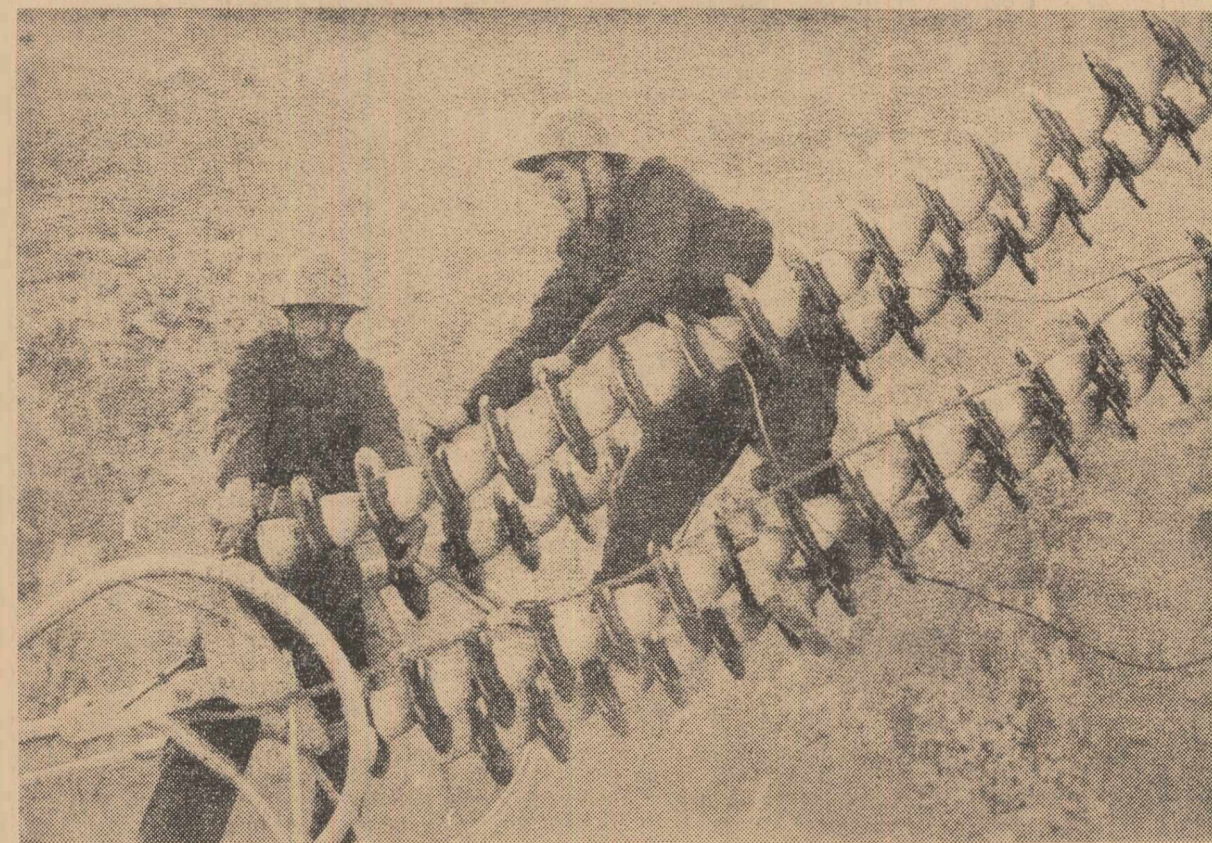
Prezența liniilor, suspendați între cer și pămînt, lîpind conductorii între stîlpii de înaltă tensiune, ne-a devenit familiară. Îi întîlnim tot mai des, în zone de șes sau de munte, făurind noi și noi conducte aeriene prin care energia electrică este transportată de la un capăt de zare la alt capăt de zare. Instantaneul surprins de fotoreporter înfățișează doi asemenea îndrăzneți liniari de pe șantierul liniei de 400 kV Luduș-Slatina
