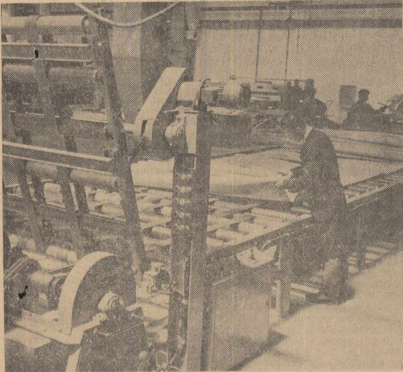
Două aspecte de la noua fabrică de placaj din cadrul C.I.L.-Sighetul Marmăției. În stînga: banda rulantă pentru transportat furnirul. În dreapta: mașina de îmbinat furnir
