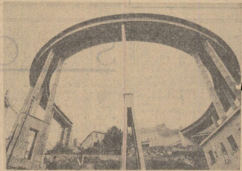
Porțiunea „Belvedere”, care face parte din viaductul ridicat peste riul Polcevera, aflat în construcție și care constituie punctul de intersecție dintre autostrada Văii Padului și autostrada Genova-Savona. Pilonii acestui viaduct au o înălțime de 45 metri.
