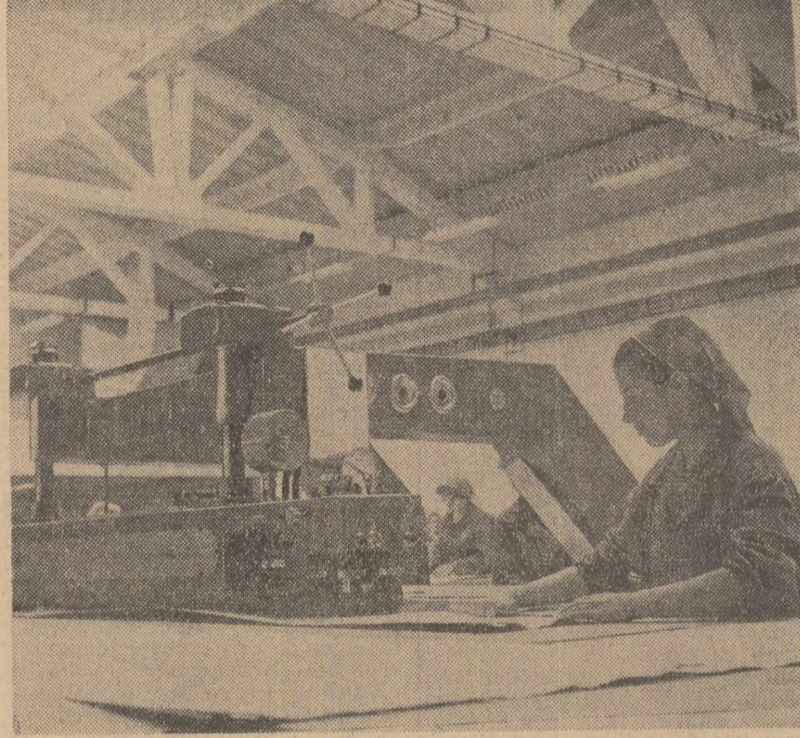
Marmăției. În stînga: banda rulantă pentru transportat furnirul. În dreapta: mașina de îmbinat furnir
