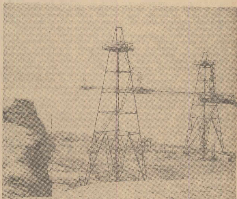
În peninsula Celeken (U.R.S.S.) crește rapid extracția de țiței și gaze. Această regiune a Turkmenei devine un mare centru al industriei petroliere a Uniunii Sovietice. Una din particularitățile schelelor petroliere din peninsula Celeken constă în aceea că turlele de foraj, la fel ca cele de pe malul cr. Jalt al Caspicei, pornesc departe în mare. În ultima vreme, în peninsula Celeken se dezvoltă cu succes forajul maritim. A început construcția unei noi uzine, care va produce blocuri de temelie pentru instalațiile de foraj în lărgul mării. Blocurile metalice formează insule, dintre care una a și apărut deasupra mării, la cîțiva kilometri de Celeken. Fotografia înfățișează estacada petrolieră de foraj maritim de pe peninsula Celeken
