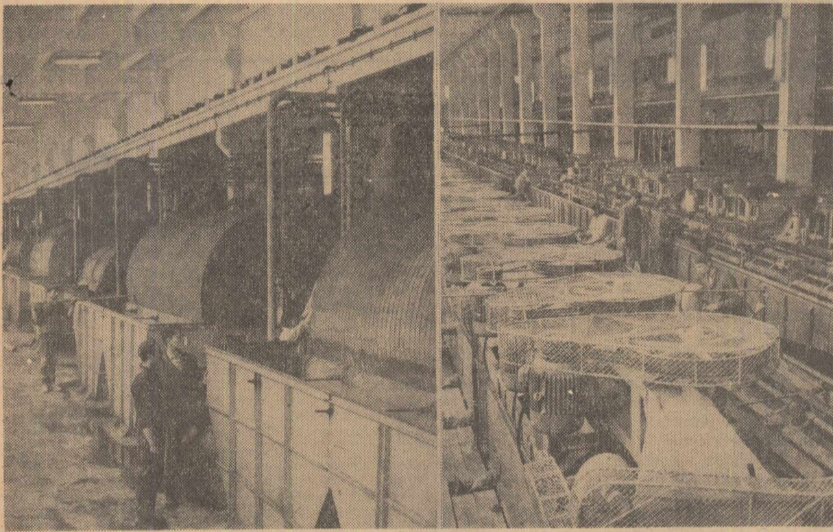
Complexul minier Leșul Ursului. În stânga: Hala îngroșătoarelor și a pompelor de vid ale stației de flotație. În dreapta: Hala celulelor de flotație
