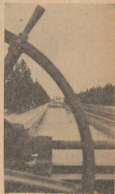
Instalațiile de la Arcuda fac parte din complexul de lucrări pentru asigurarea alimentării cu apă a Bucureștilor. La Arcuda, apa este captată din râul Dimbovița, decantată, filtrată, dezincercată și apoi redată ca apă potabilă. În cîșeu: Vedere exterioră a filtrelor lento
