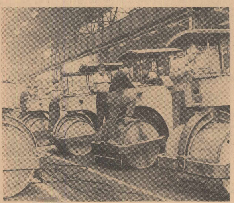
Uzina de utilaj greu „Progresul” din Braila produce diferite utilaje grele necesare șantierelor de construcții, printre care și rulouri compresoare. Colectivul secției în care se produc rulouri compresoare s-a angajat să dea peste plan, în cinstea celui de-al IV-lea Congres al Partidului, 10 bucăți rulouri compresoare. Pînă în prezent, ei au și realizat 4 dintre acestea. În clișeu: Echipa condusă de Ion Danciu sub supravegherea maestrului Dumitru Ciurea, lucrează la montarea unui nou lot de rulouri compresoare Foto: NICU VASILE
