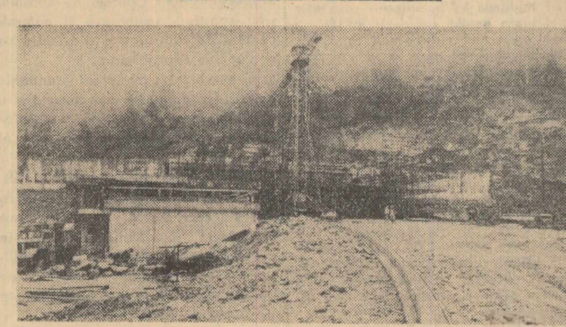
Lucrările de construcție a celui mai lung tunel din lume, tunelul-șosea Mont Blanc, cu o lungime de aproximativ 7 mile și jumătate, se află într-un stadiu avansat. În fotografie: aspect de pe unul din șantierul noului tunel
