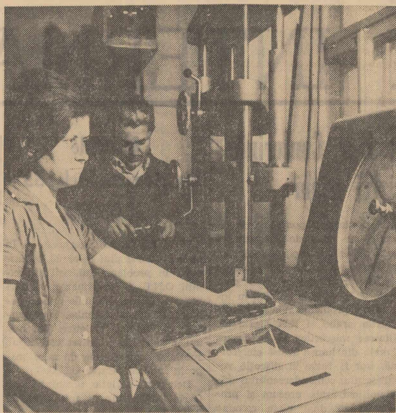
Ing. Al. Oprea împreună cu laboranta Vasileca Oleanu din cadrul laboratorului de încercări mecanice al Uzinelor „23 August”, stabilesc cu ajutorul mașinii de tracțiune de douăzeci de tone rezistența la rupere a unor materiale.
