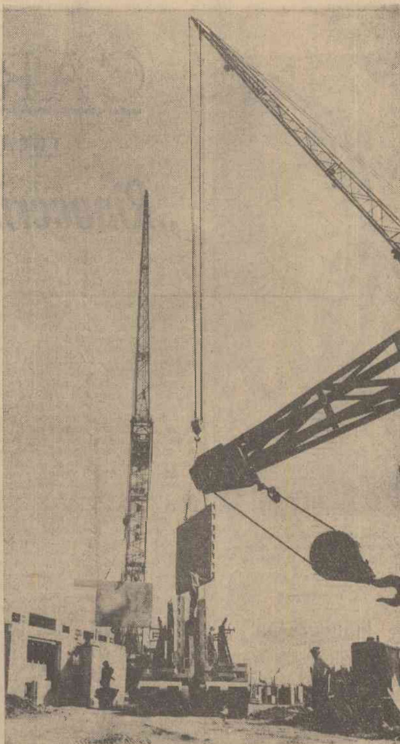
Pe bulevardul Armata poporului din capitală, s-a deschis recent un front de lucru pentru construirea a 960 de apartamente. În prezent, la două blocuri a început montarea panourilor mari prefabricate, iar la alte 6 blocuri sînt în curs săpăturile fundațiilor. În cîșeu: Aspect de pe șantierul nr. 2 al I.C.M.-5
