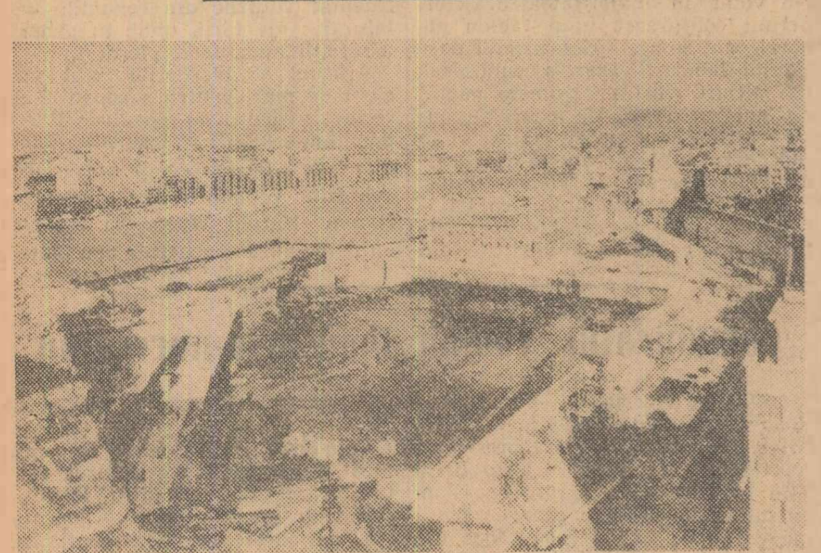
Amenajarea unui tunel sub vechiul port francez Marsilia este o mare operațiune care va transforma în cițiva ani aspectul marelui oraș mediteranean. Lung de 600 de m, tunelul submarin, destinat să lege cartierele Fort Saint-Jean și Fort Saint-Nicolas, va permite un trafic de 60.000 vehicule pe zi. Fotografia înfățișează un aspect de pe șantierul de construcții al tunelului.
