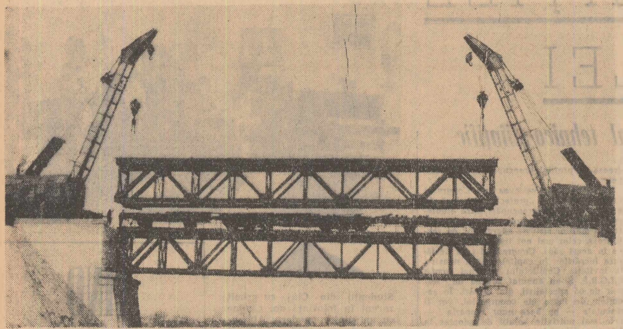
Vă prezentăm în imagine fotografică o raționalizare. Este vorba de o recentă lucrare executată de întreprinderea de construcții transporturi Craiova care a lansat cu ajutorul a două macarale de mare tonaj un nou tablier metalic la podul Bratcov-Roșiori de Vede. Raționalizarea constă în înlocuirea metodei de construcție element cu element a tablauerii la fața locului, cu metoda montării sale separat la sol și apoi lansarea. În acest fel s-a scutit timpul de lucru, nu s-a întrerupt circulația, s-a micșorat efortul fizic al muncitorilor, realizându-se totodată economii la prețul de cost în valoare de aproximativ 60 000 lei.
