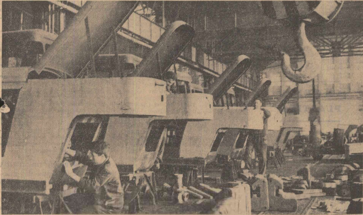
Ca furnizor, Uzina „Progresul” din Brăila, participă la realizarea a numeroase produse. În același timp la utilajele pe care le execută colaborează cu alte zeci de întreprinderi. În cliseu: Unul din aceste utilaje: un nou lot de rulouri compresoare în stadiul de montaj. Foto: AGERPRES
